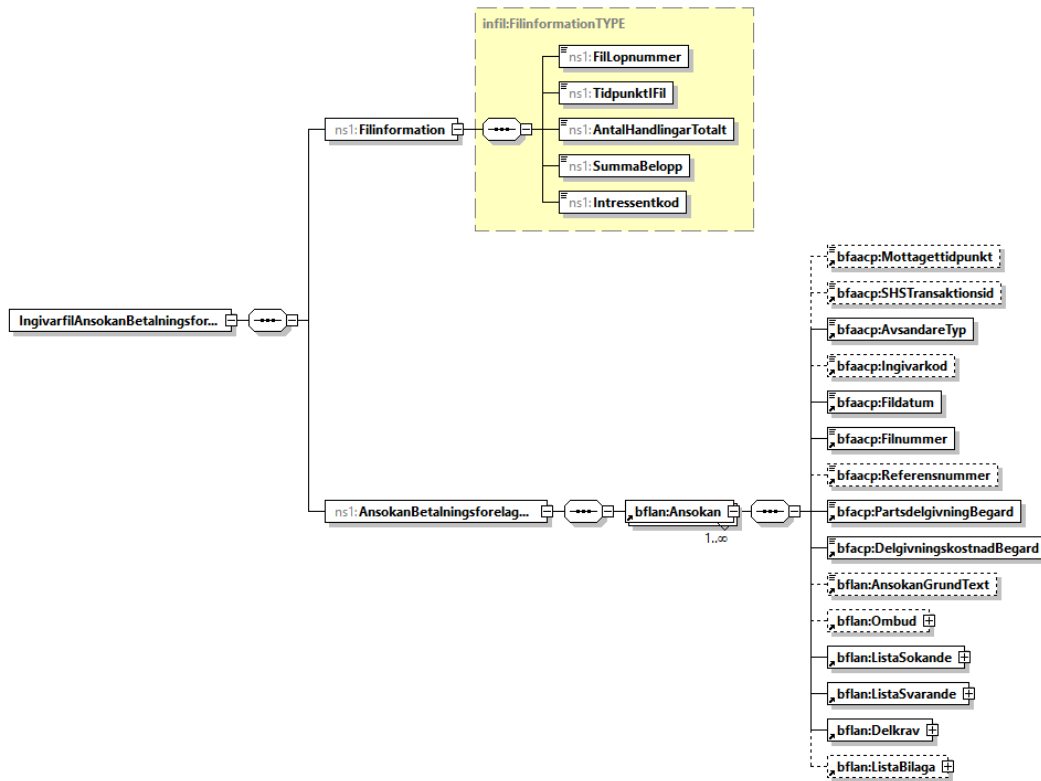
Figur 2 - Transaktionsfilens struktur
