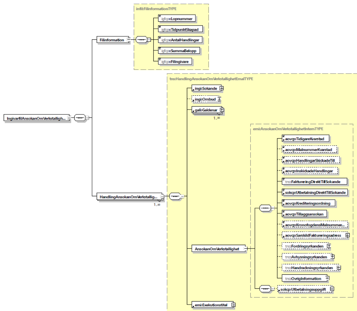
Figur 2 - Transaktionsfilens struktur
