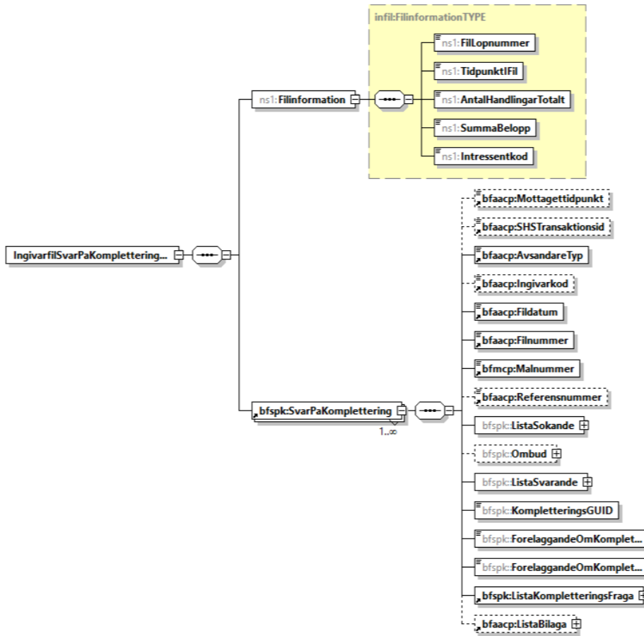
Figur 2 - Transaktionsfilens struktur
