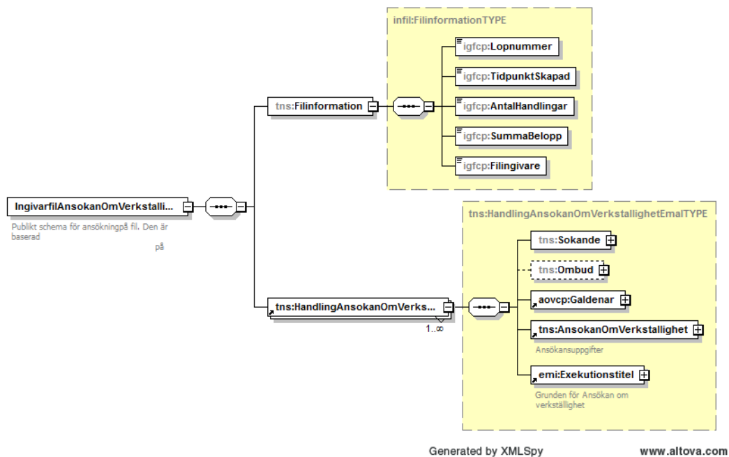
Figur 2 - Transaktionsfilens struktur
