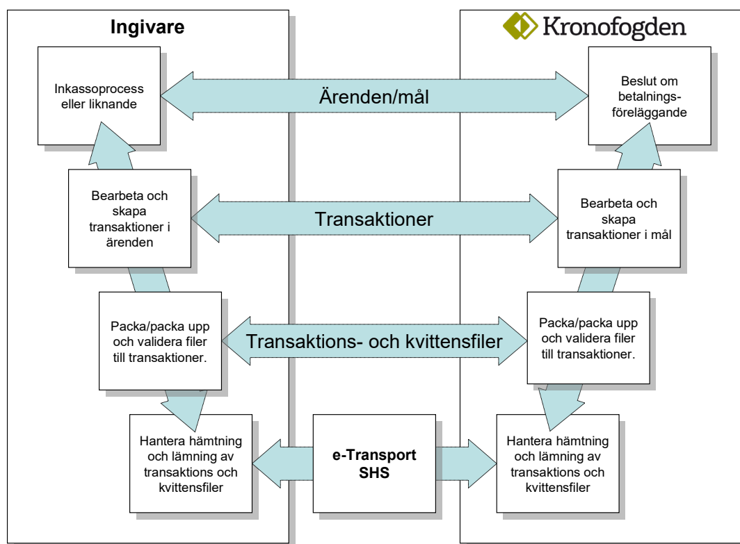
Figur 2 - Kommunikationsmodell
